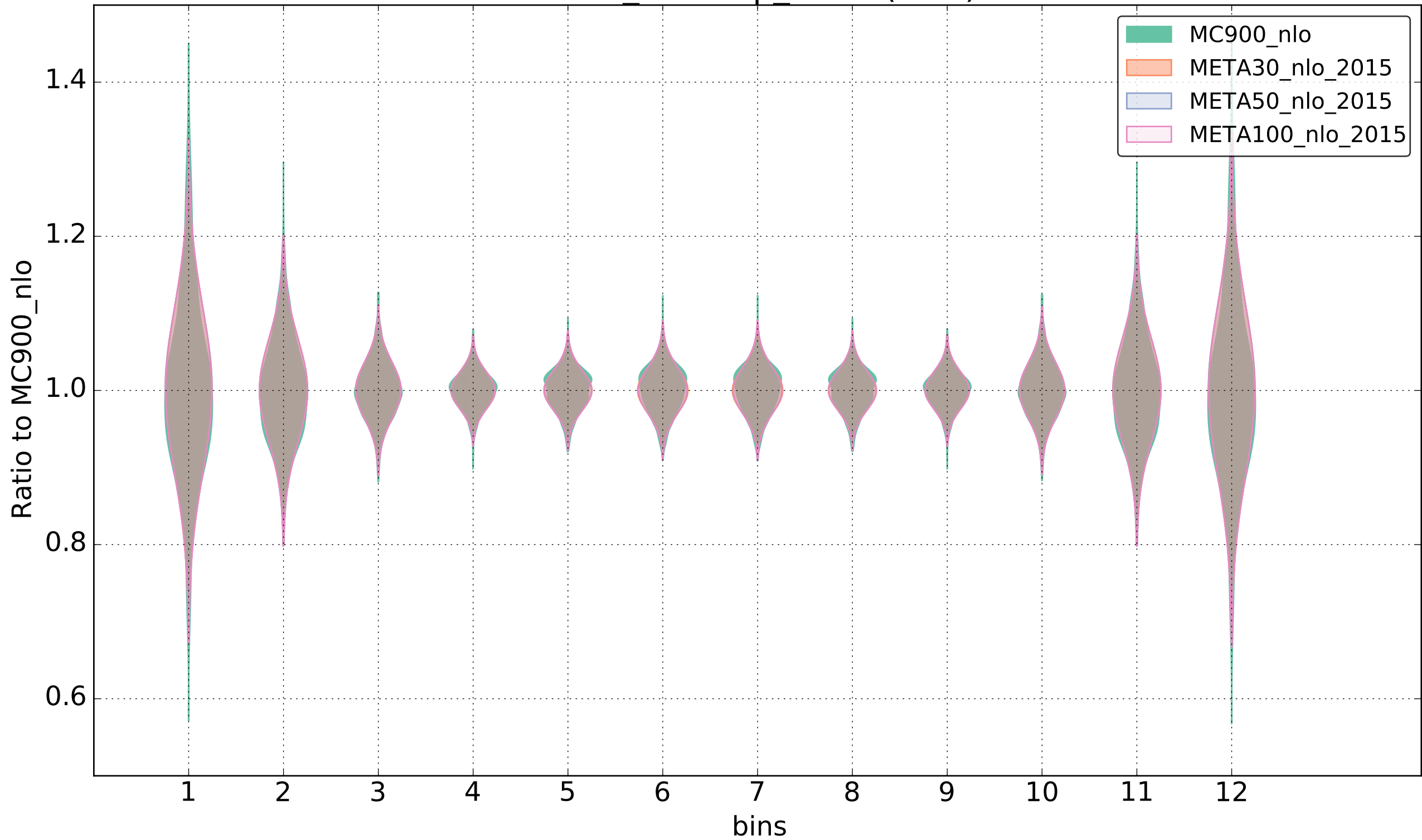
ttbar_ttbarap_13tev(NLO)
