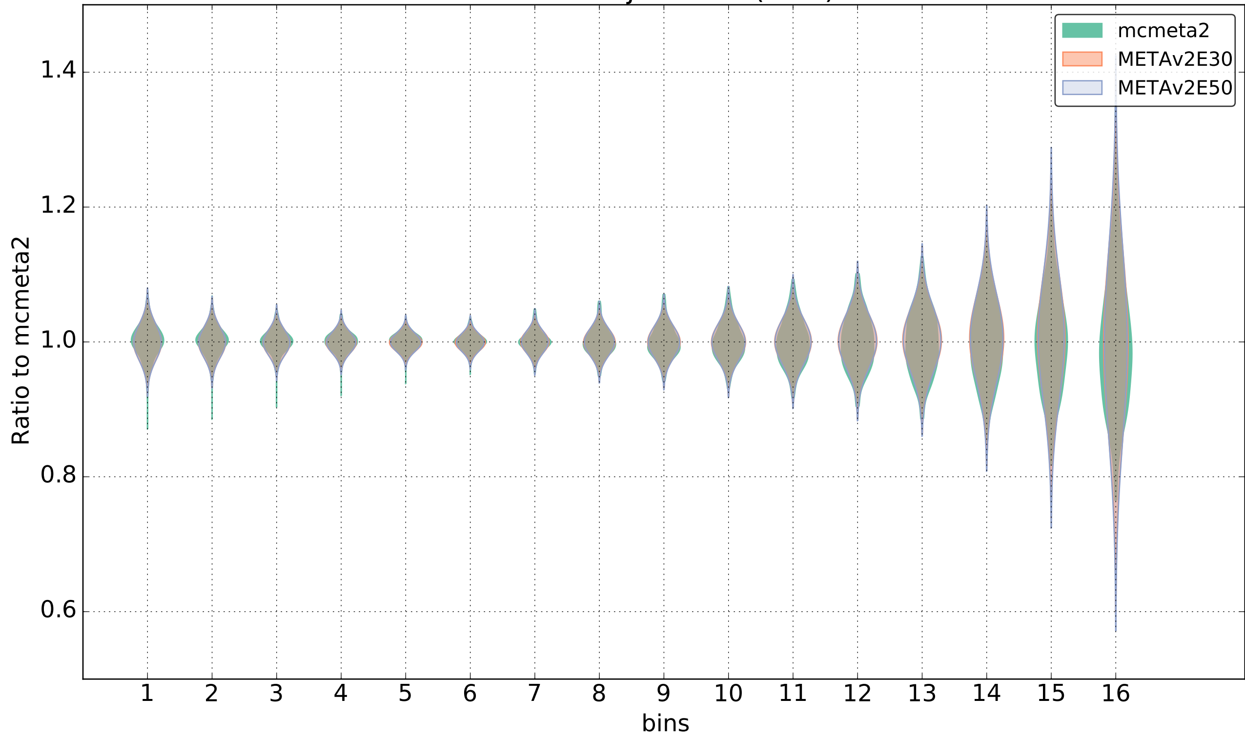
atlas-incljets-eta3(NLO)
