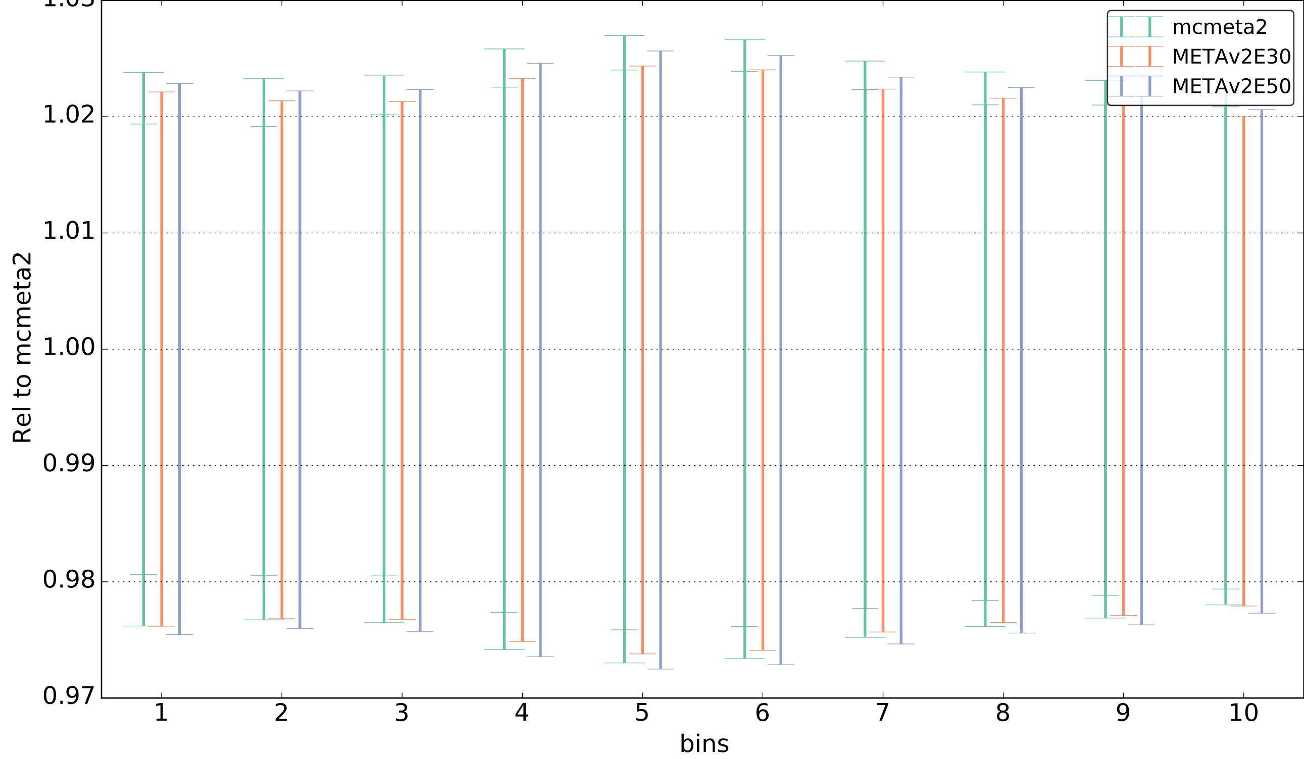
z_lplminvmas 13tev(NLO)
