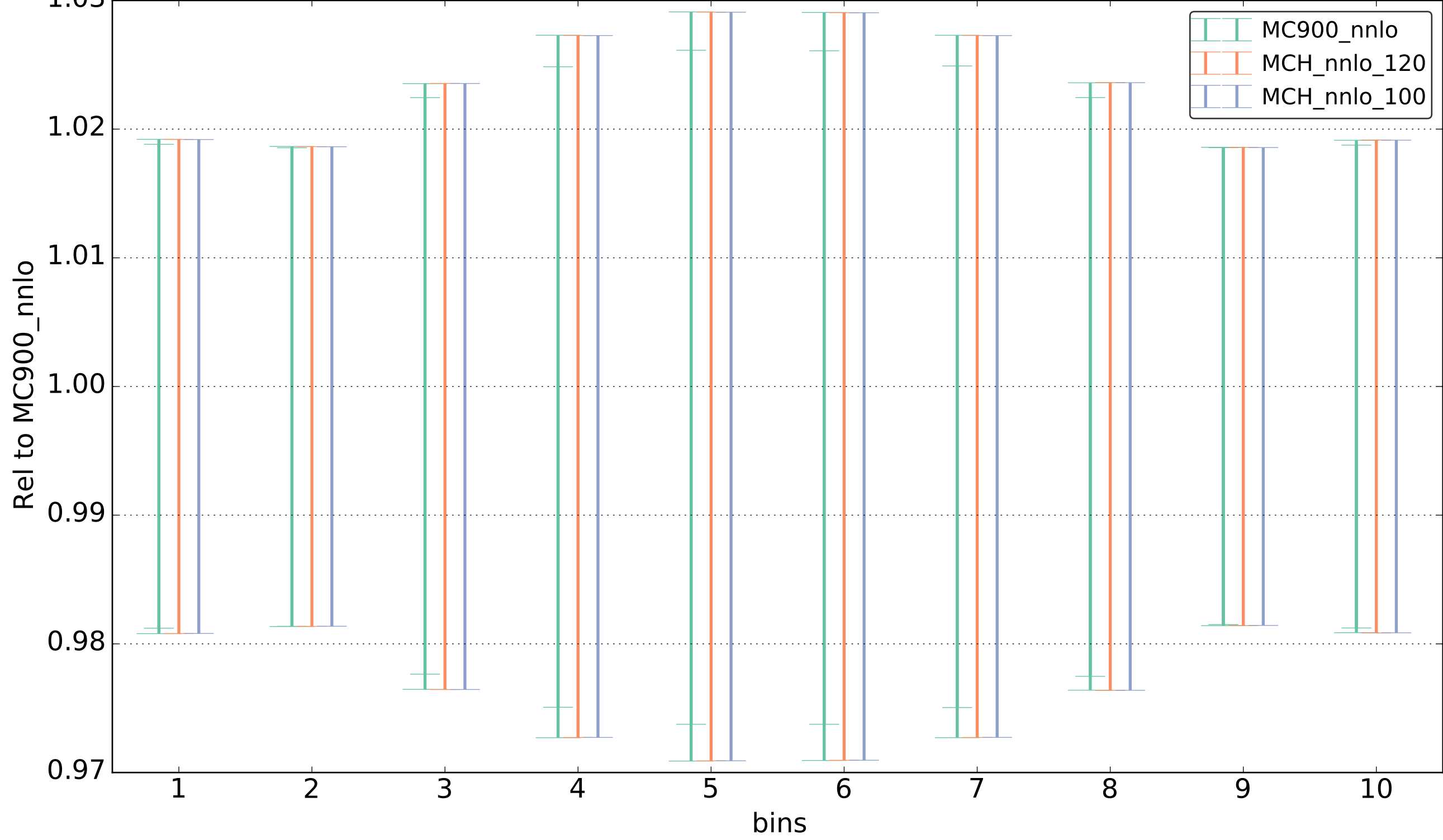
ggH_y_13tev(NLO)
