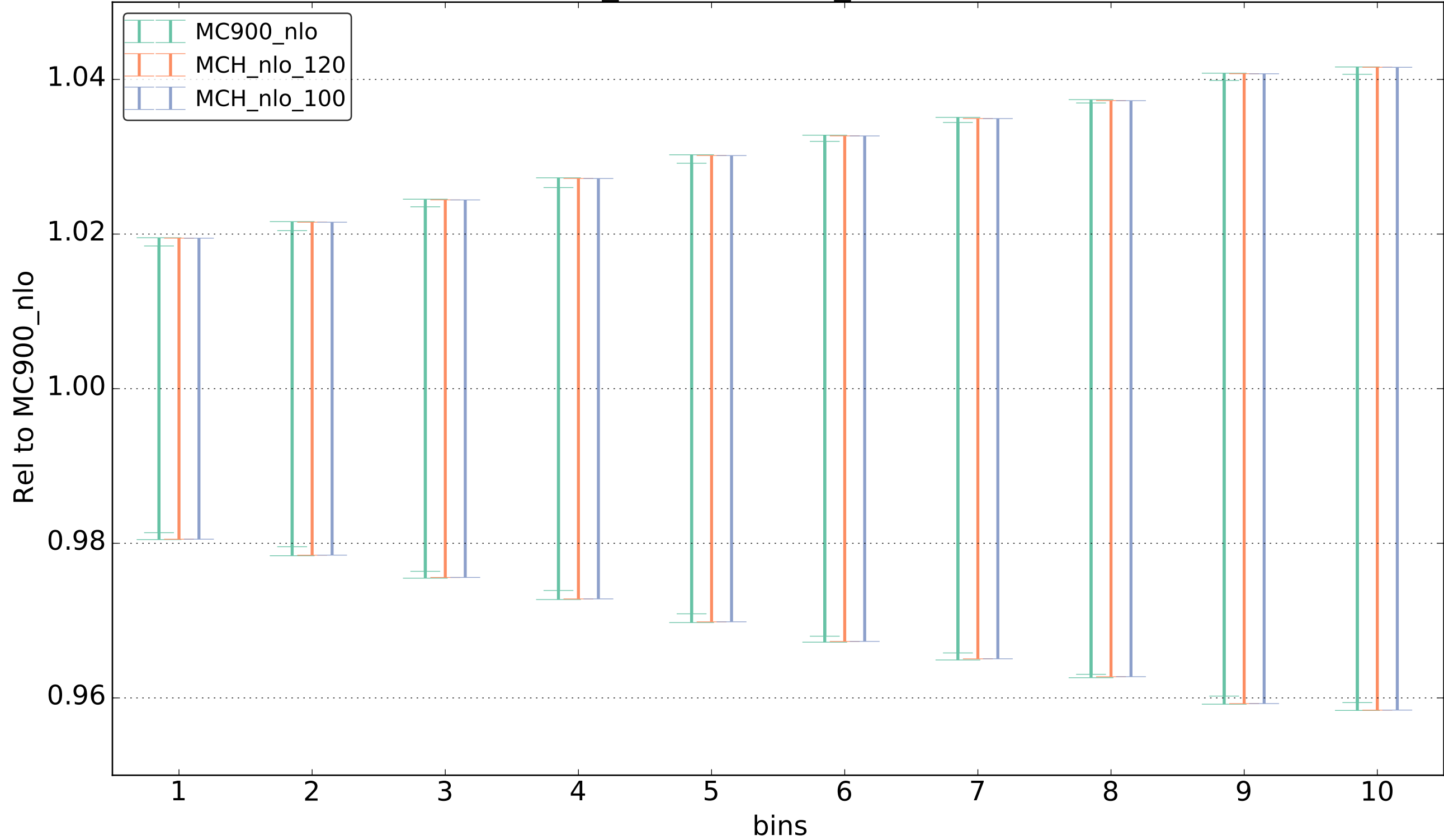
ttbar ttbarinvmass 13tev(NLO)
