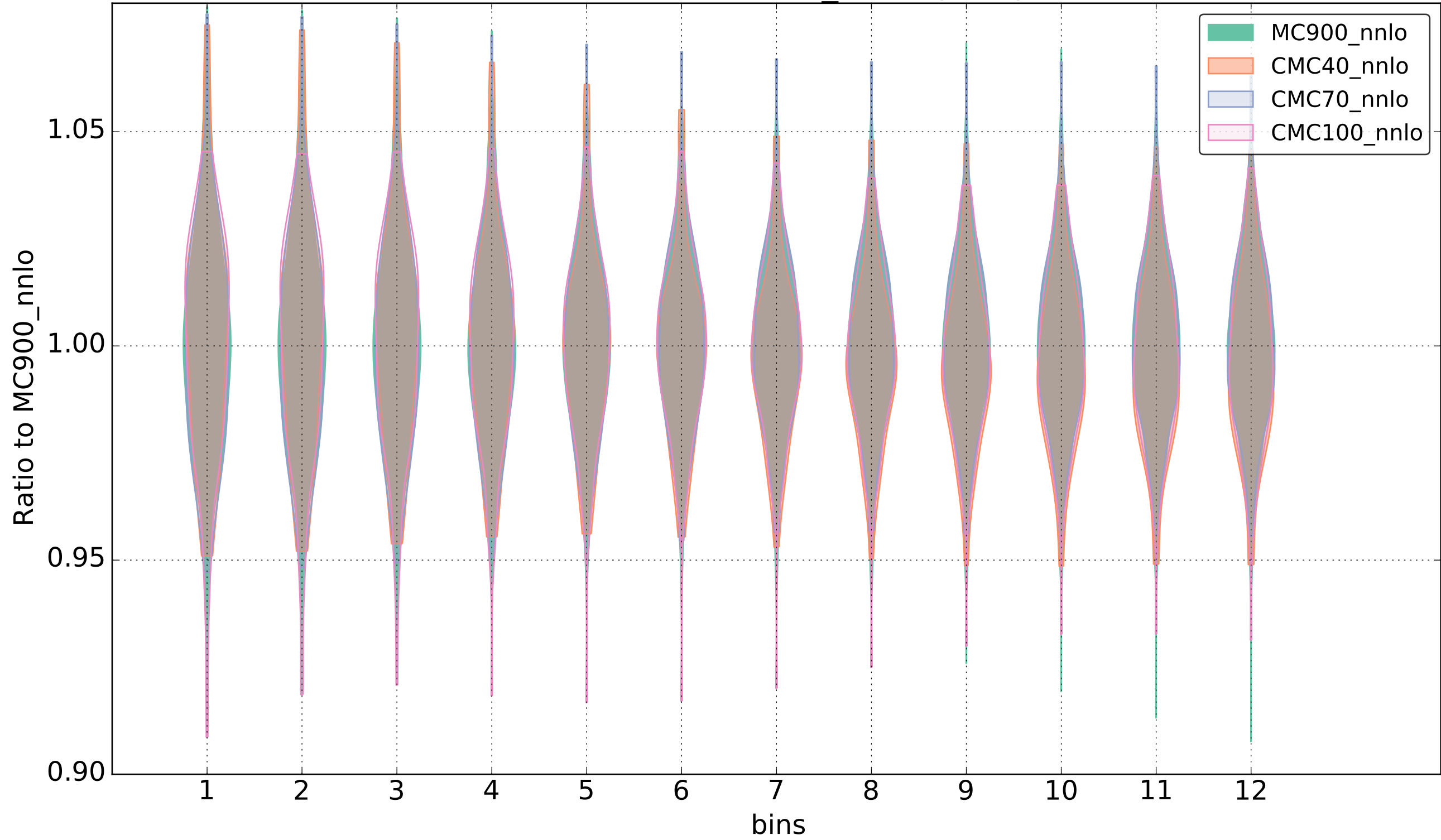
CMSDY2D11-bin6_eta34(NLO)
