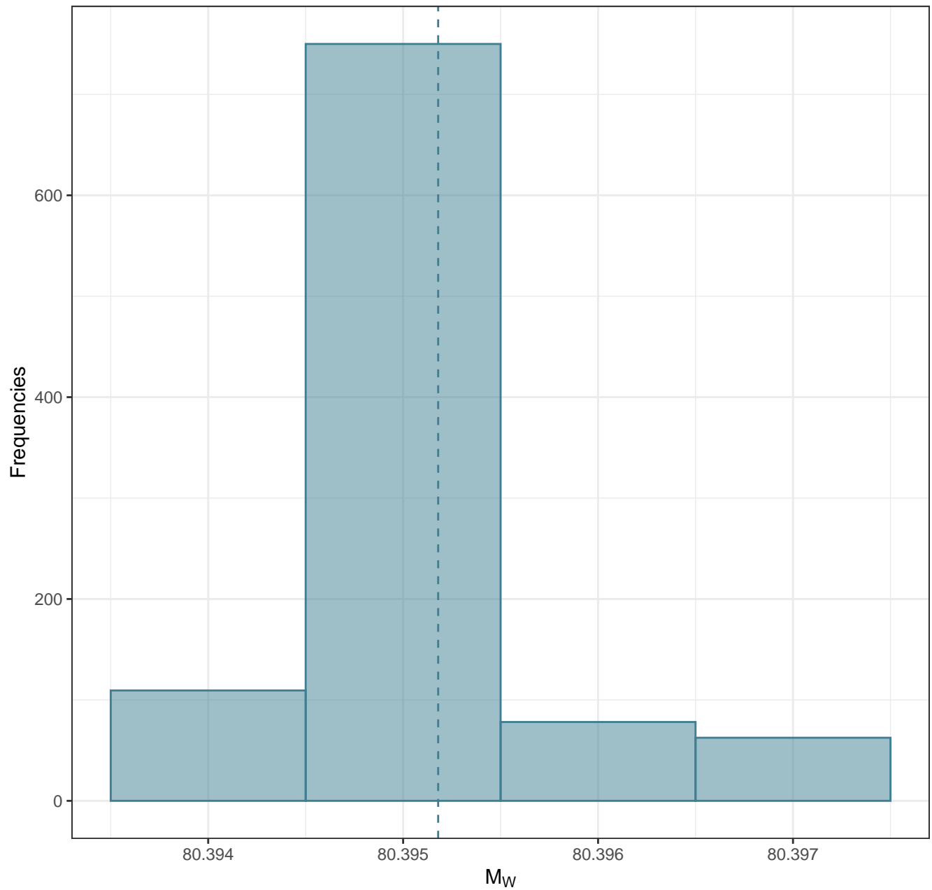
Mw Distr. 80.394 MSHT20nnlo_as118
