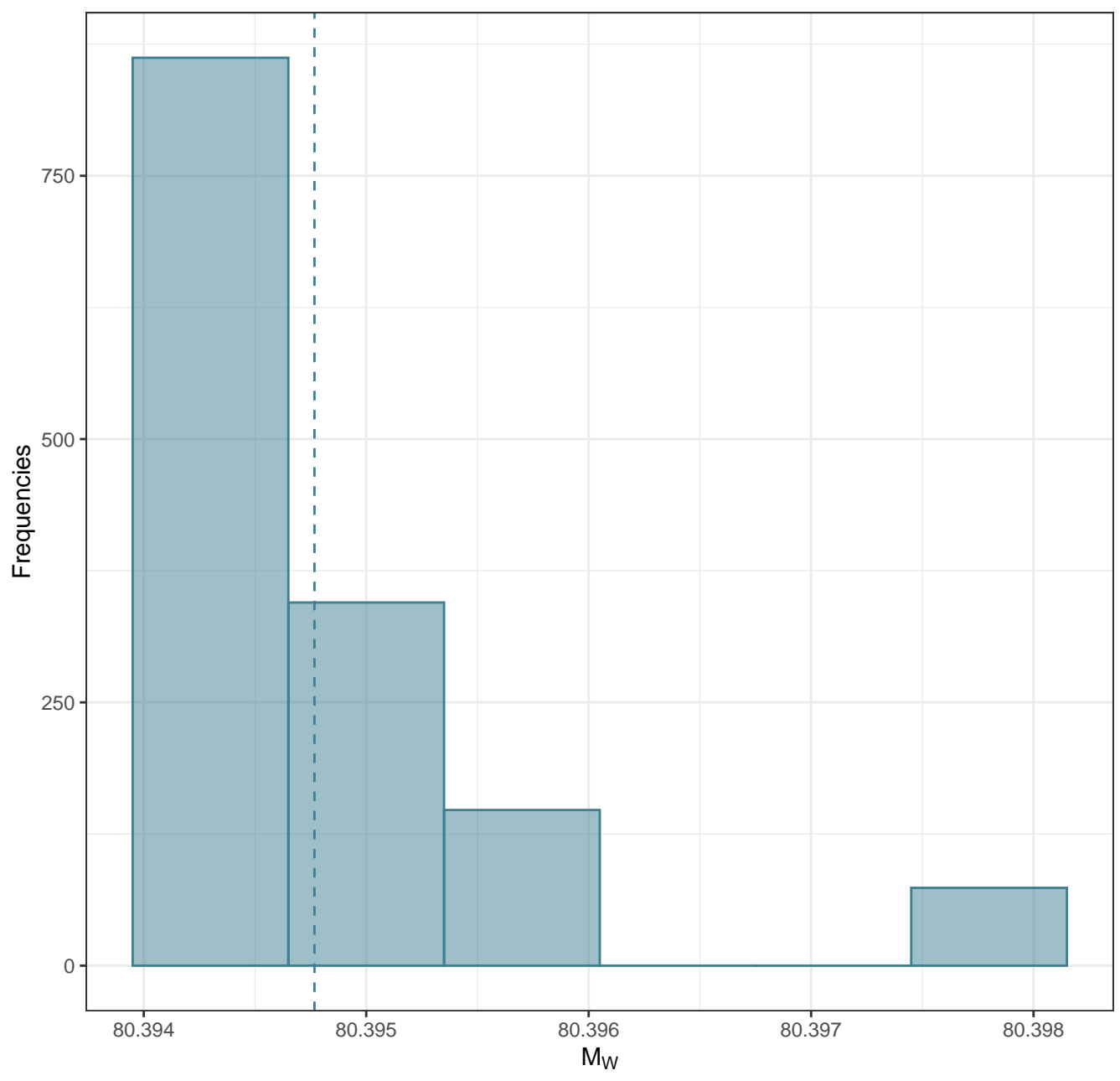
Mw Distr. 80.394 CT18NNLO
