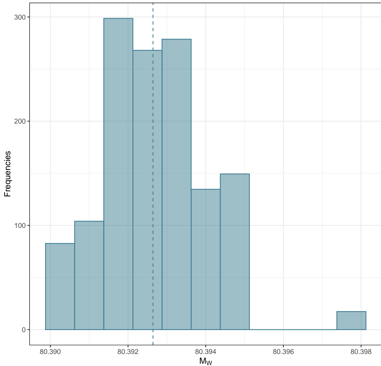
Mw Distr. 80.394 210715-n3fit-1000-001
