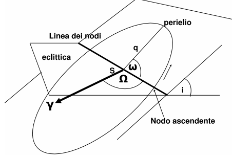
FIGURE 5. Gli elementi orbitali.
