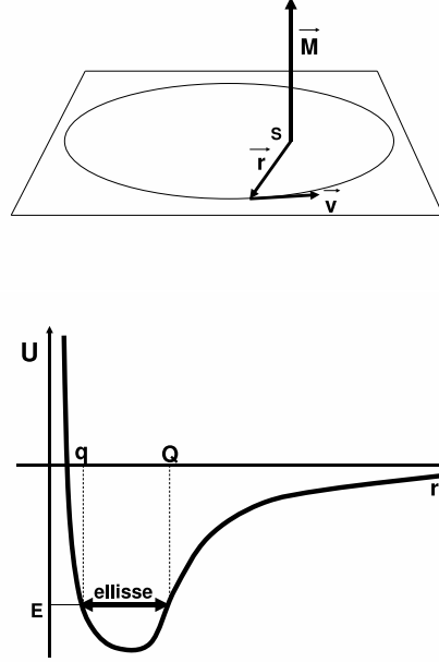
FIGURE 3. a) Il momento angolare orbitale è un vettore ortogonale ai vettori posizione e velocità. b) L'energia potenziale per il moto radiale (potenziale gravitazionale e centrifugo). Fissando l'energia totale si hanno una (iperbole e parabola) o due intersezioni (ellisse). L'intersezione a distanza minore fornisce il valore di q . Nelle intersezioni la velocità radiale si annulla e si inverte.
