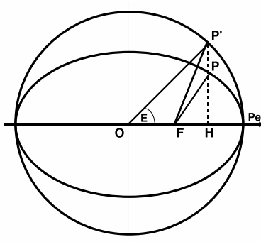
FIGURE 2. Equazione di Keplero. L'area del settore Fuoco-Perielio-punto P dell'ellisse (area spazzata dal raggio vettore) e' il riscalamento dell'area Fuoco-Perielio- punto P' sul cerchio esterno.
