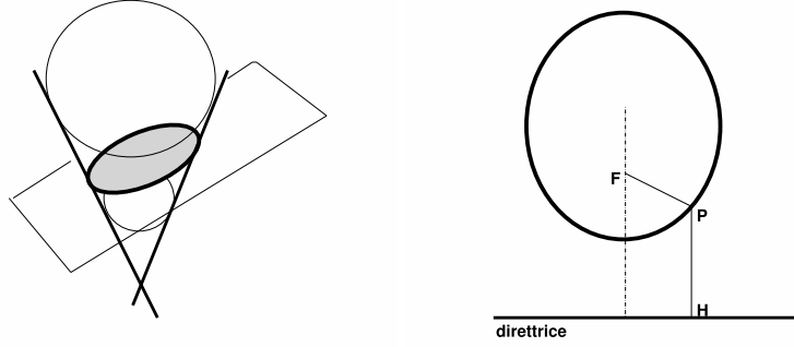
FIGURE 4. a) Un doppio cono tagliato da un piano individua due rami di iperbole (se il piano interseca entrambi i coni), una parabola (piano parallelo alla generatrice del cono), una ellisse (il piano interseca solo un cono). Le sfere tangenti individuano i fuochi. b) Le sezioni coniche sono luoghi dei punti del piano con rapporto PF/PH = e (eccentricità).
