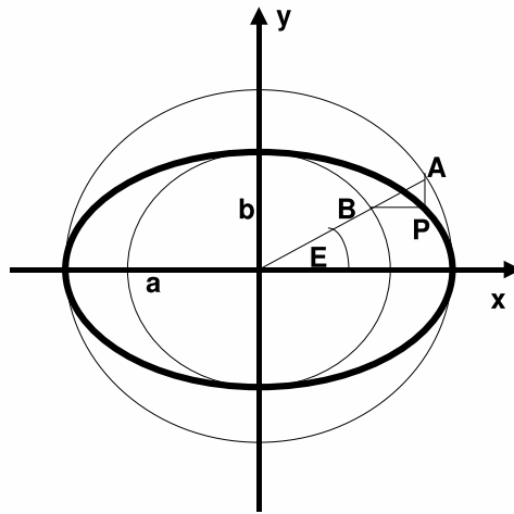
FIGURE 1. La costruzione dell'ellisse di semiassi assegnati.
